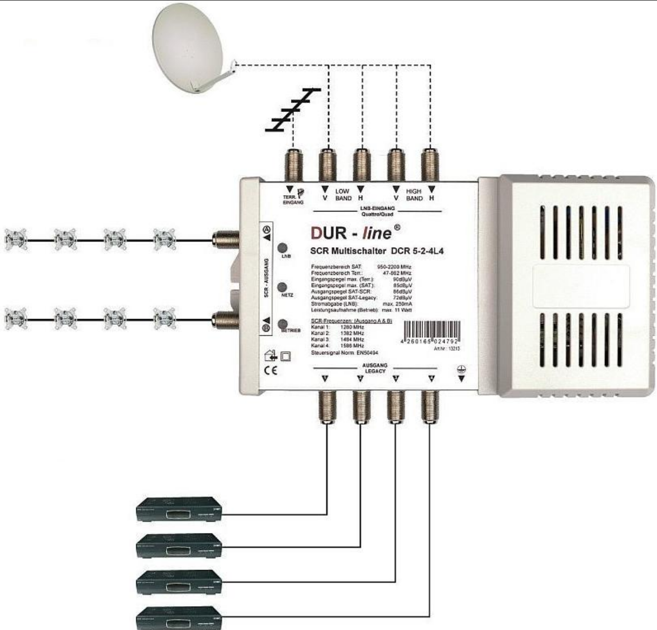
Przykład rozwiązania instalacji kaskadowej rozbudowanej o kolejny multiswitch DUR-line DCR 5-2-4L-4
